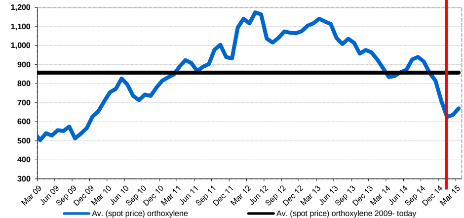
Orthoxylene
