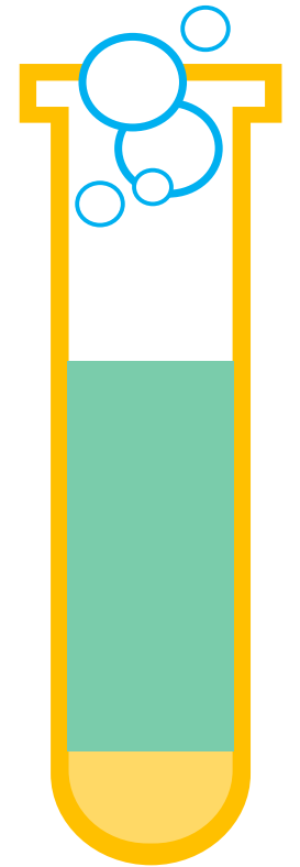
Ammonia
