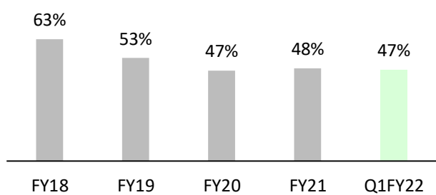
GNPA (%)
